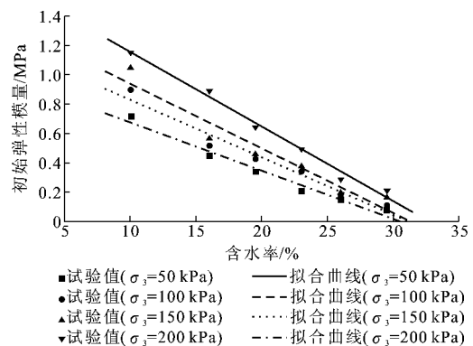
图 2 初始弹性模量随含水率的变化
