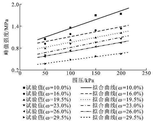
图 6 峰值强度随围压的变化
