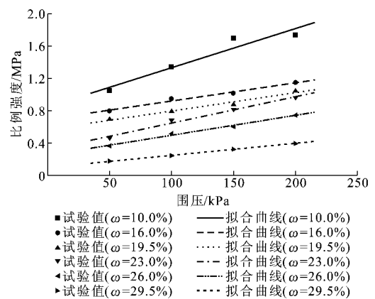
图 7 比例强度随围压的变化
