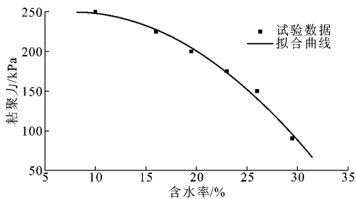
图 9 粘聚力随含水率的变化
