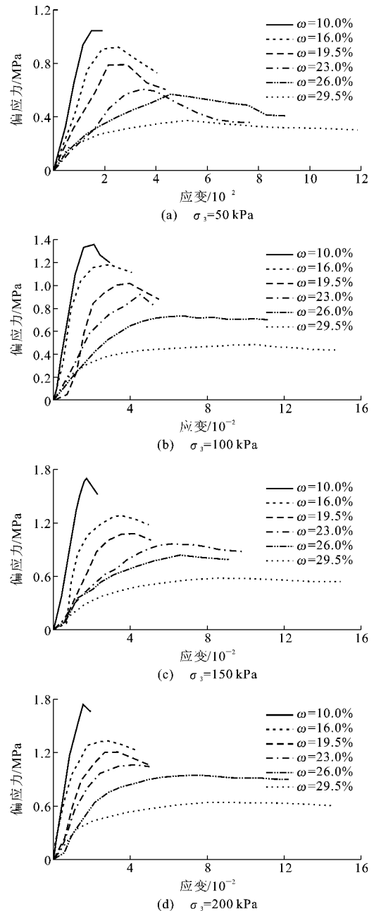
图 1 不同围压下的应力-应变关系 Fig. 1 Stress-strain Curves Under Different Confining Pressures
