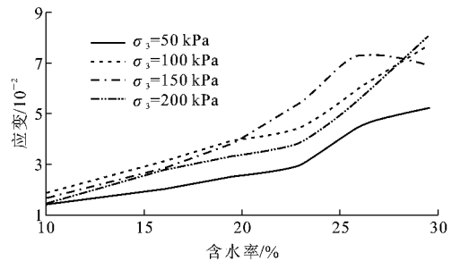
图 13 不同围压下破坏应变随含水率的变化
