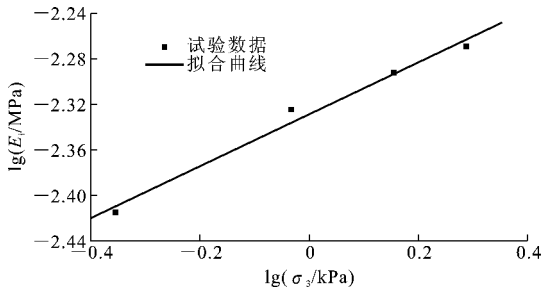
图 11 \lg(\sigma_3/\text{kPa})-\lg(E_i/\text{MPa}) 关系
