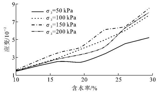
图 12 峰值强度时应变随含水率的变化
