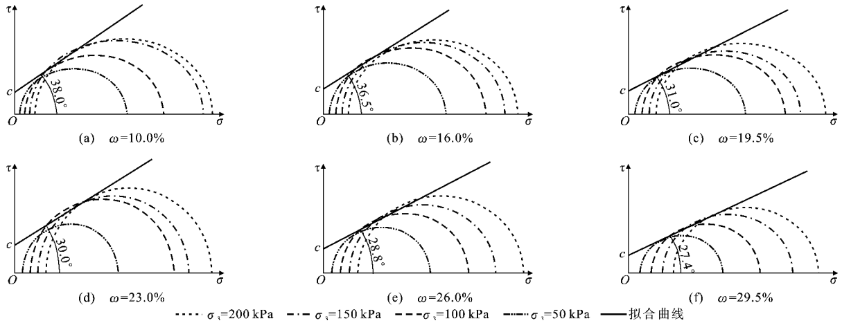
图 8 灰土的抗剪强度包络线
