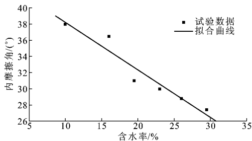
图 10 内摩擦角随含水率的变化
