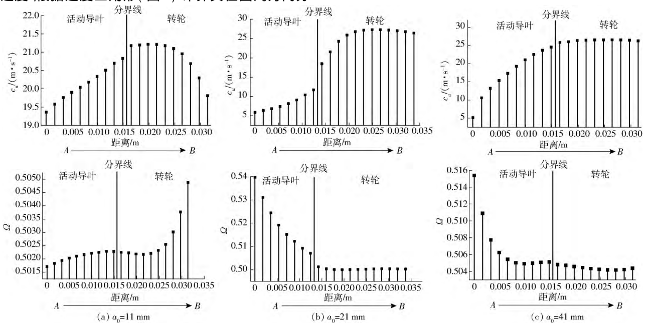
图 8 c_u 、 \Omega 分布
