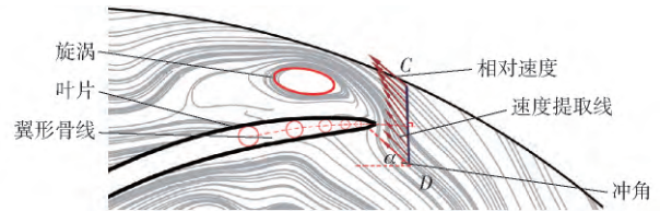
图 11 叶片进口冲角示意图
