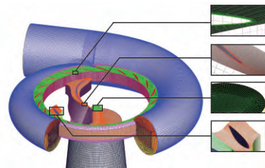
图2 局部网格示意图
