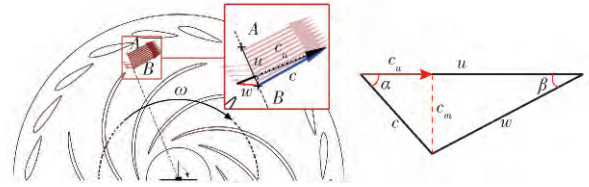
图 7 径向速度提取图以及速度三角形
