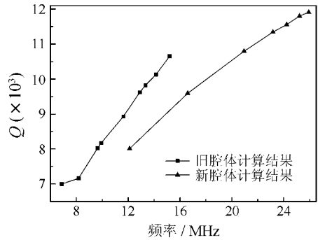
图 3 新旧腔体 Q 值频率关系曲线
