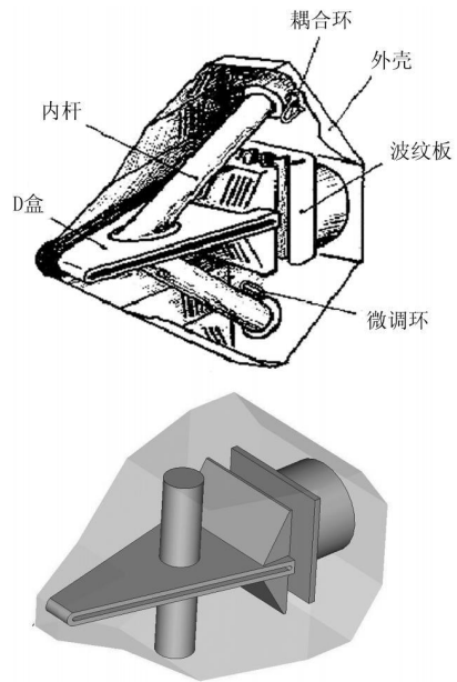
图 1 SSC 新旧两种腔体结构比较
