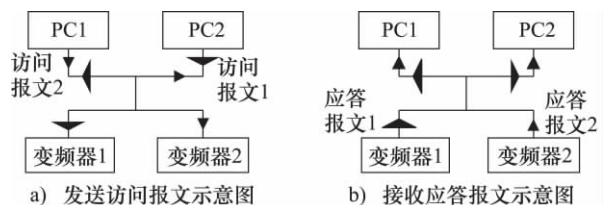
图6 多主多从式RS-485通信原理示意图
