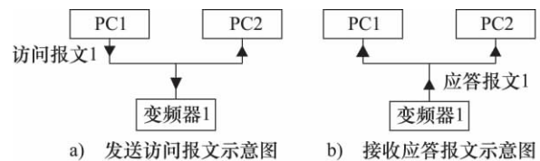
图5 多主多从式RS-485通信原理示意图
