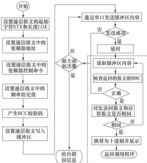
图 7 RS-485 多主多从结构通信流程图
