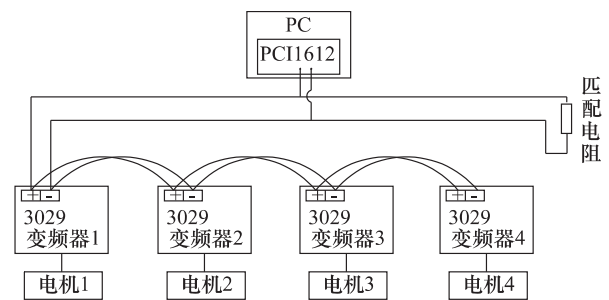
图 2 一主多从式 RS-485 变频调速系统图
