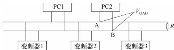
图4 多主节点RS-485短路结构示意图
