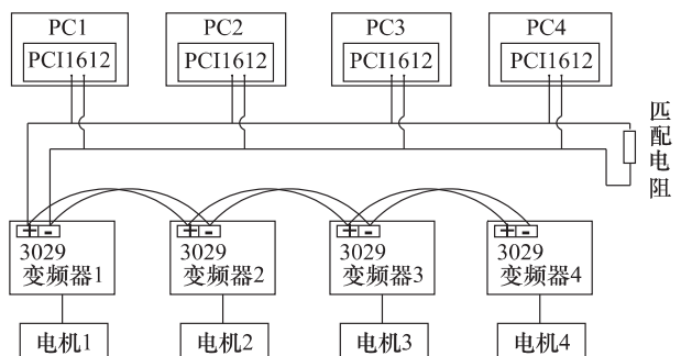
图 3 多主多从式 RS-485 变频调速系统图
