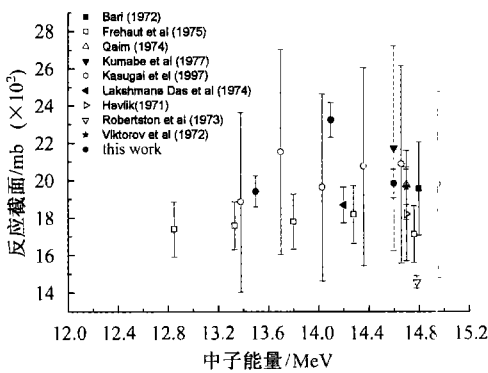
图 1 ^{160}\text{Gd}(n, 2n)^{159}\text{Gd} 的反应截面
