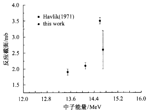
图 2 ^{158}\text{Gd}(n, p)^{158}\text{Eu} 的反应截面
