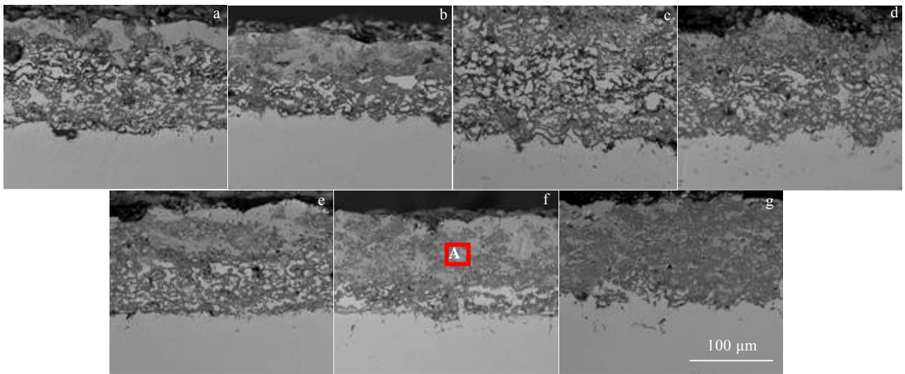
图 5 NiCoCrAlY 真空扩散涂层在 1050 下不同氧化时长的微观形貌
