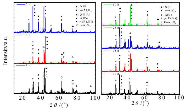
图 8 1050 ℃ 时 NiCoCrAlY 真空扩散涂层不同氧化时长的 XRD 图谱
