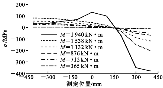
图 13 外钢管纵向应力
