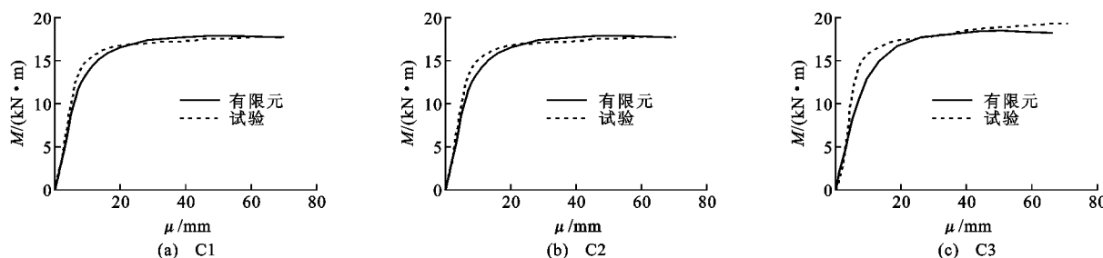
图3 中空夹层圆钢管混凝土构件弯矩-跨中挠度(M-μ)曲线
