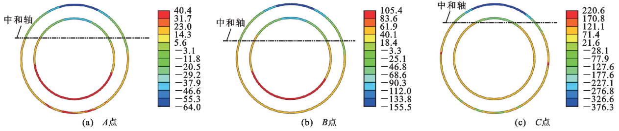
图 10 节点处内外钢管纵向应力(单位:MPa)
