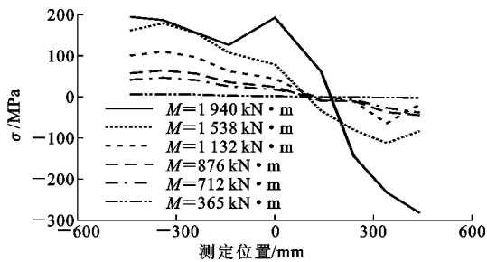
图 14 外加劲肋纵向应力
