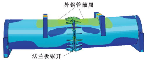
图 6 内外法兰节点破坏形态
