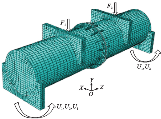
图 5 加载方式和网格划分示意图
