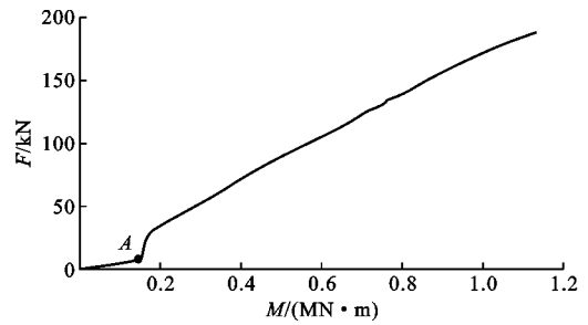
图 12 最大螺栓拉力-弯矩曲线
