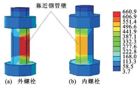
图 9 内外法兰板底端最大螺栓屈服应力云图(单位:MPa)
