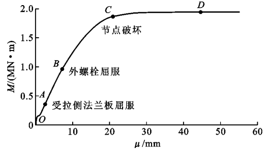
图 7 M-\mu 曲线
